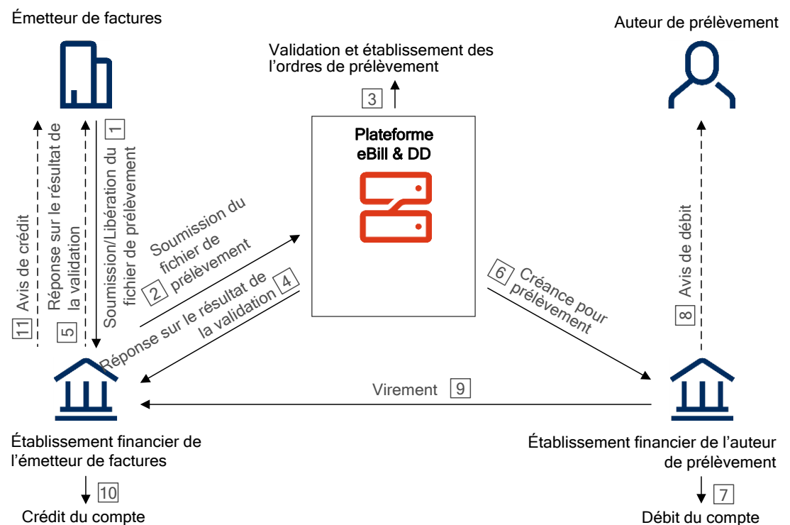
Illustration 6: Processus de soumission par l'émetteur de factures via son établissement financier
